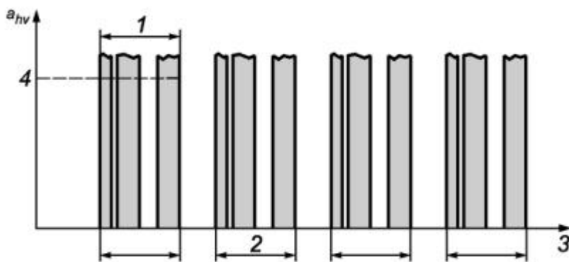
1 - длительность измерений; 2 - время воздействия вибрации (в данном случае, общее время использования инструмента); 3 - время; 4 - a_{hv, measured}
