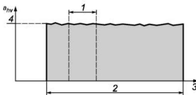
Рисунок Е.1 - Продолжительные измерения при непрерывной работе ручной машины
