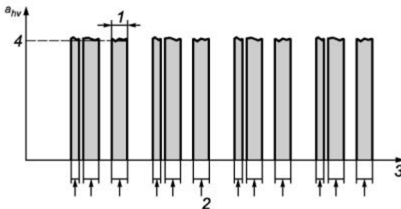
1 - длительность измерений; 2 - время воздействия вибрации (в данном случае, общее время работы инструмента); 3 - время; 4 - a_{nv, measured}
