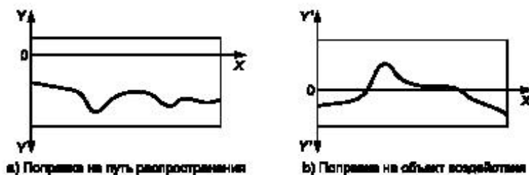
Рисунок 3 — Элементы модели источника вибрации
