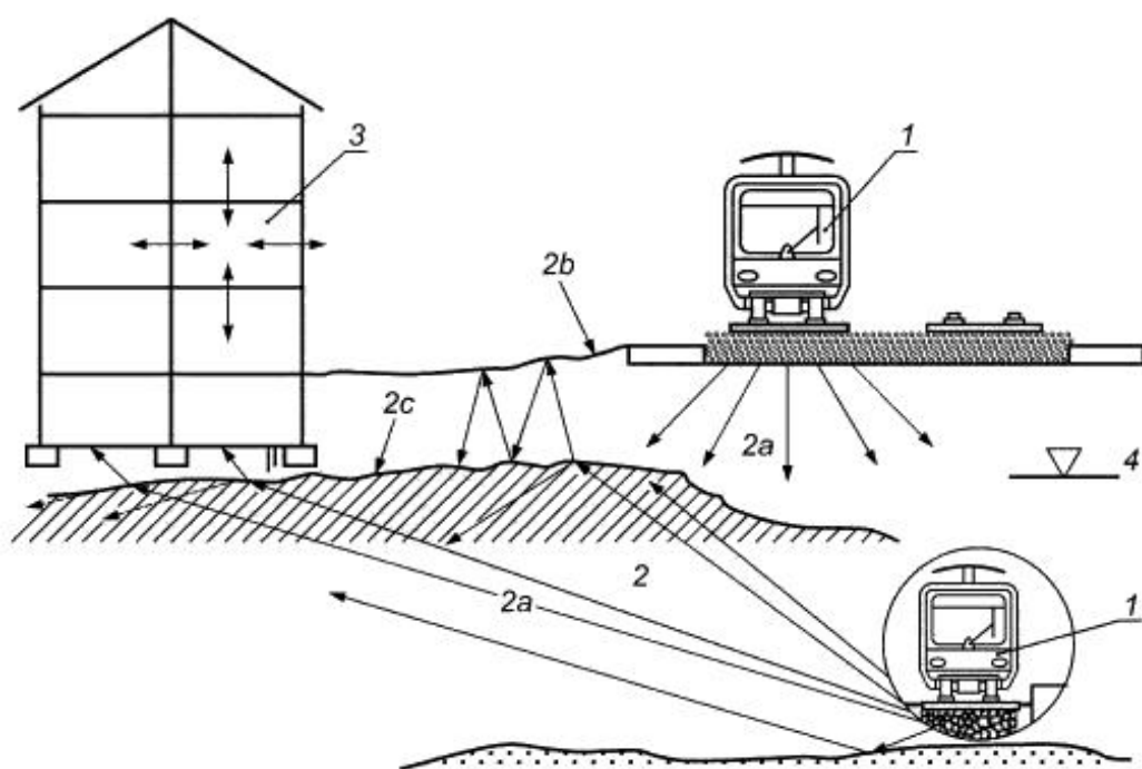
1 — источник вибрации; 2 — путь распространения (2a — волны внутри тела, сжатия, сдвига; 2b — поверхностные волны Рэлея, Лява; 2c — волны на границе сред: Стоунли); 3 — объект воздействия (вибрация, переизлученный шум); 4 — поверхность грунтовых вод
