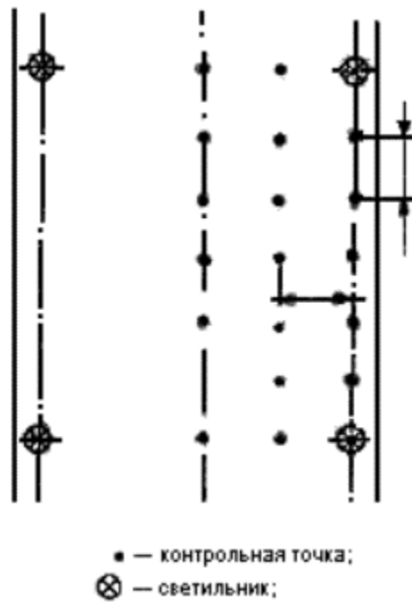
Рисунок А6 - Расположение контрольных точек при измерении средней освещенности улиц при двухстороннем шахматном расположении светильников
