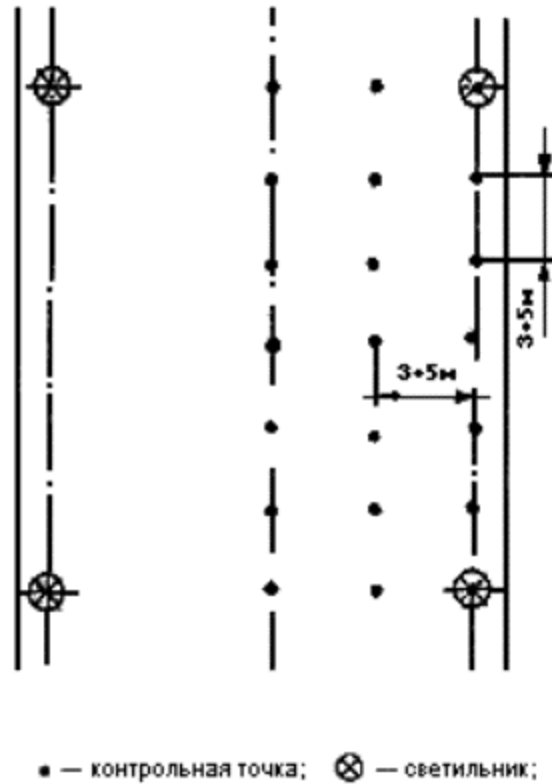
Рисунок А5 - Расположение контрольных точек при измерении средней освещенности улиц при двухстороннем прямоугольном расположении светильников
