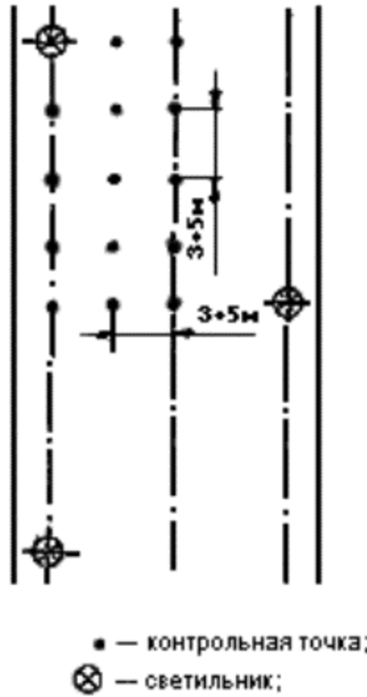
Рисунок А6 - Расположение контрольных точек при измерении средней освещенности улиц при двухстороннем шахматном расположении светильников
